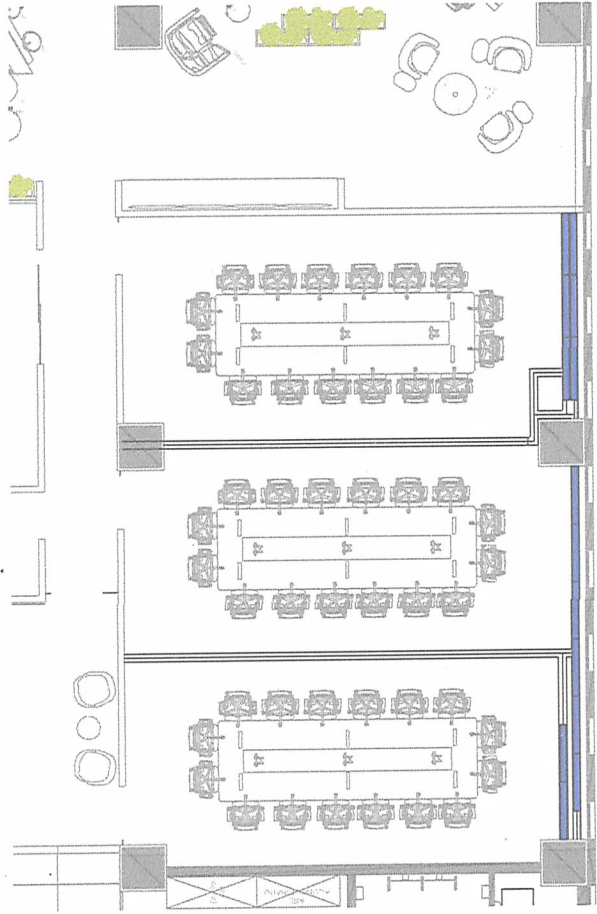
1 PLANTA MUROS MOVILES 1:50
