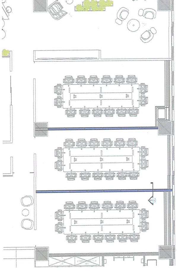
2 PLANTA MUROS MOVILES 1:50
