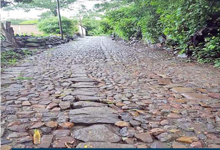
— Empedrado calle Belisario Domínguez en la Delegación de Tepec. Inversión: $9,000.00 Alcance: 420 metros cuadrados.
