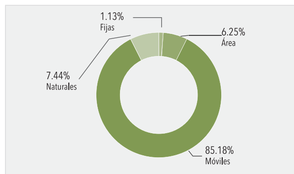
Gráfico 2.2. Porcentaje de emisiones a la atmósfera por tipo de fuente
