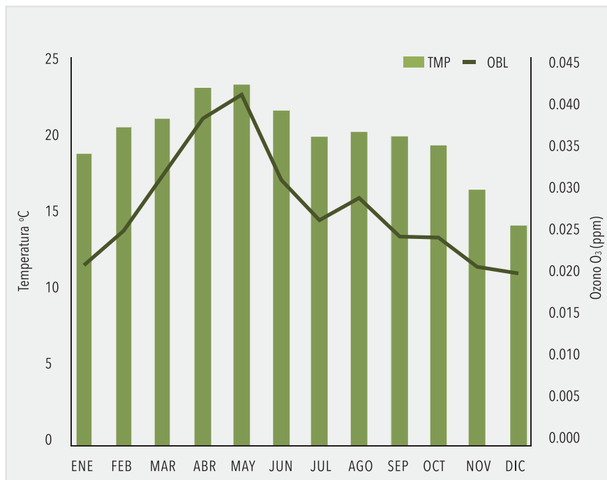
Gráfico 2.3. Comportamiento del Ozono en el transcurso del año
