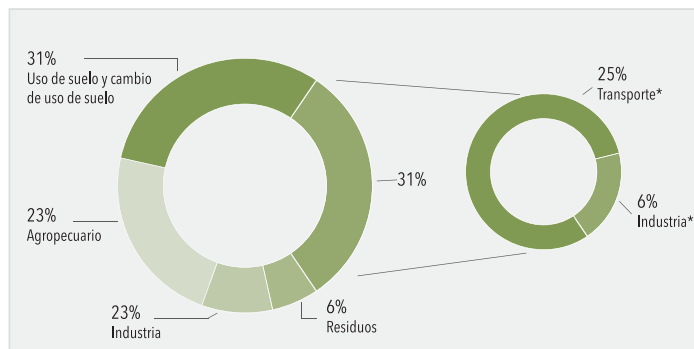
Gráfico 3.3. Porcentaje de emisiones contaminantes por sector en Jalisco
