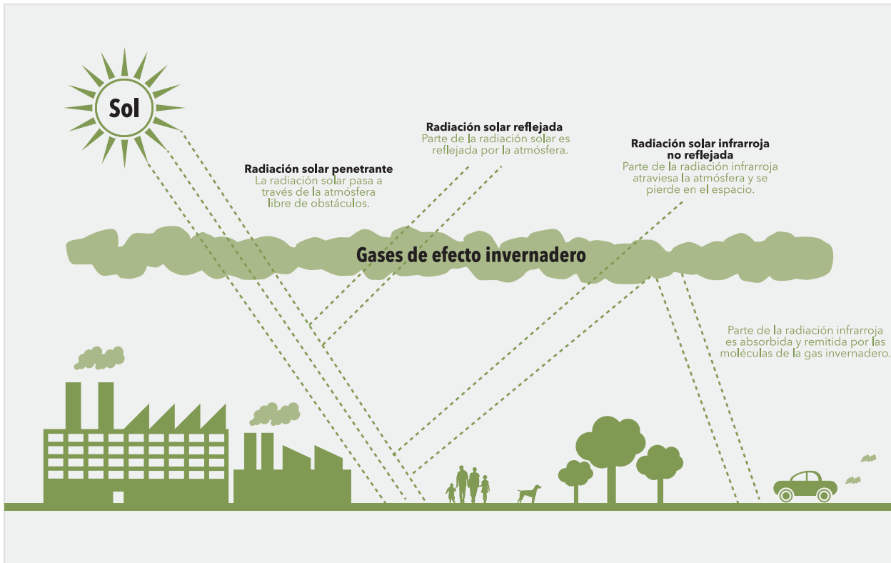
Gráfico 3.1 Infografía de efecto invernadero
