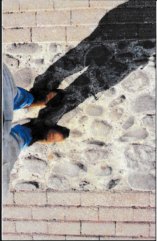
EMPEDRADO CONVENCIONAL COLocado SOBRE UNA CAMA DE T-9 Y LECHERILADO CON MORTERO CEMENTO
