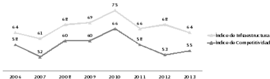
Gráfica 1.1 Posición de México en el Índice de Infraestructura y de Competitividad, 2006-2013 (Posición mundial)
