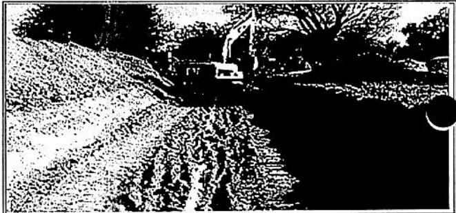
Excavación en la ubicación donde convergen los colectores sanitarios de Buenavista, el Bajío, Orilla del Agua y Torrecillas.
